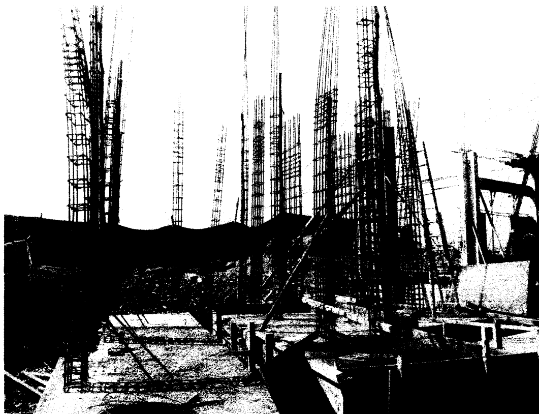
Foto N° 10: Vaciado de concreto en zapatas, e izaje de acero de columnas.
