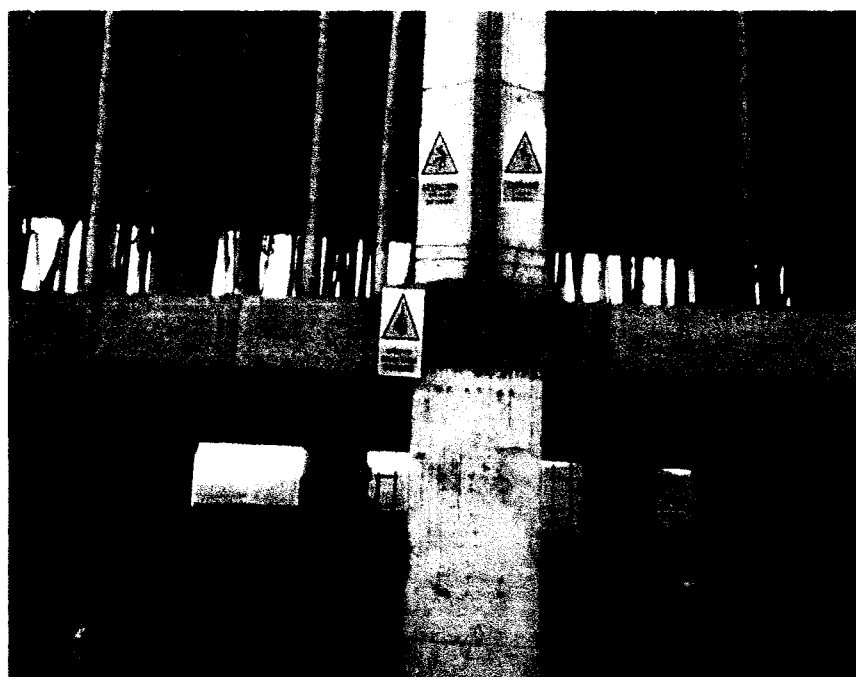
Foto 10: delimitación del área con avisos preventivos de caídas de objetos, peligro con la carga suspendida, caídas
