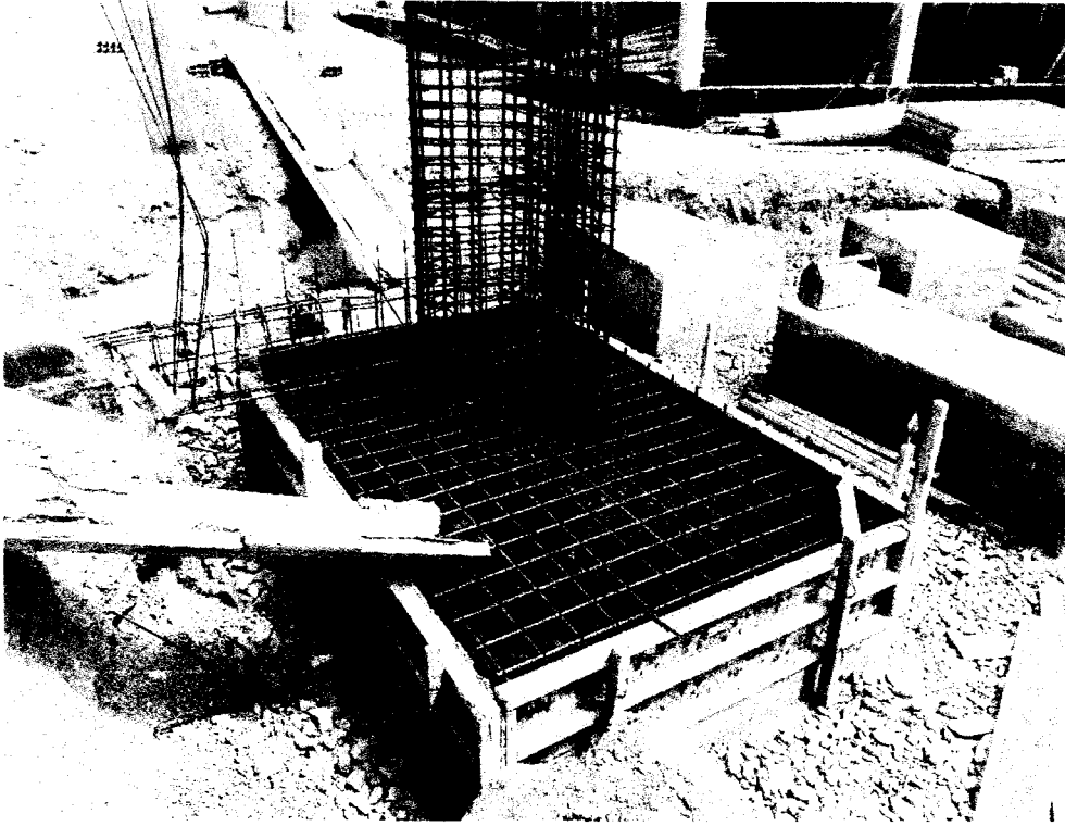
FOTO N° 03: Colocado de acero en zapatas y columnas, Tareas previas.
