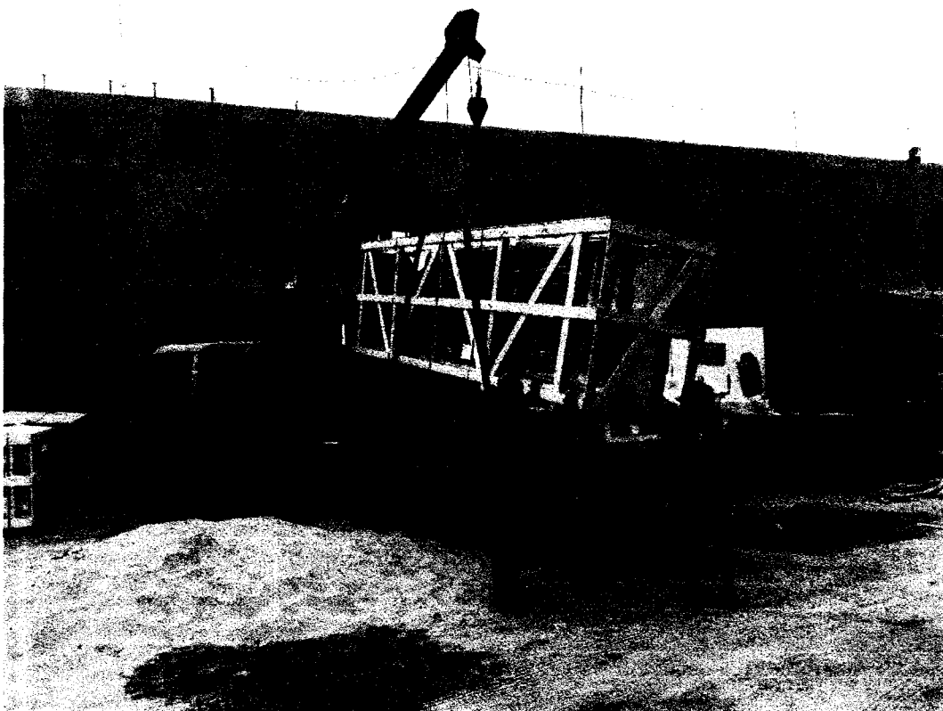
Foto N° 18: Almacenamiento del equipamiento en obra.
